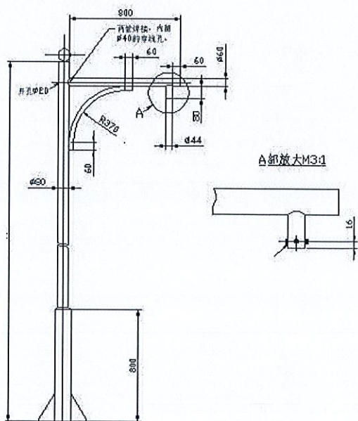
立杆结构图
